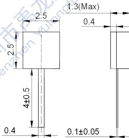
其它未注公差: ±0.25mm 尺寸单位: mm
