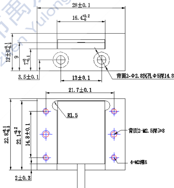
尺寸单位: mm
