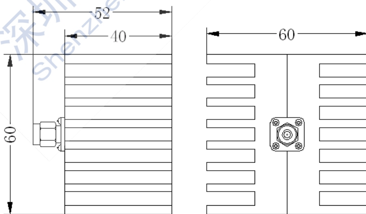
尺寸单位: mm 外形尺寸公差: \pm 2\%
